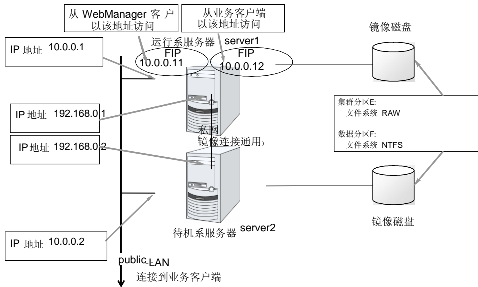
图 2-6 使用镜像磁盘时的集群环境示例
