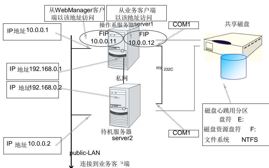
图 2-4 使用共享磁盘时的集群环境示例
