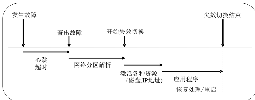
图 2-3 失效切换的时间表
