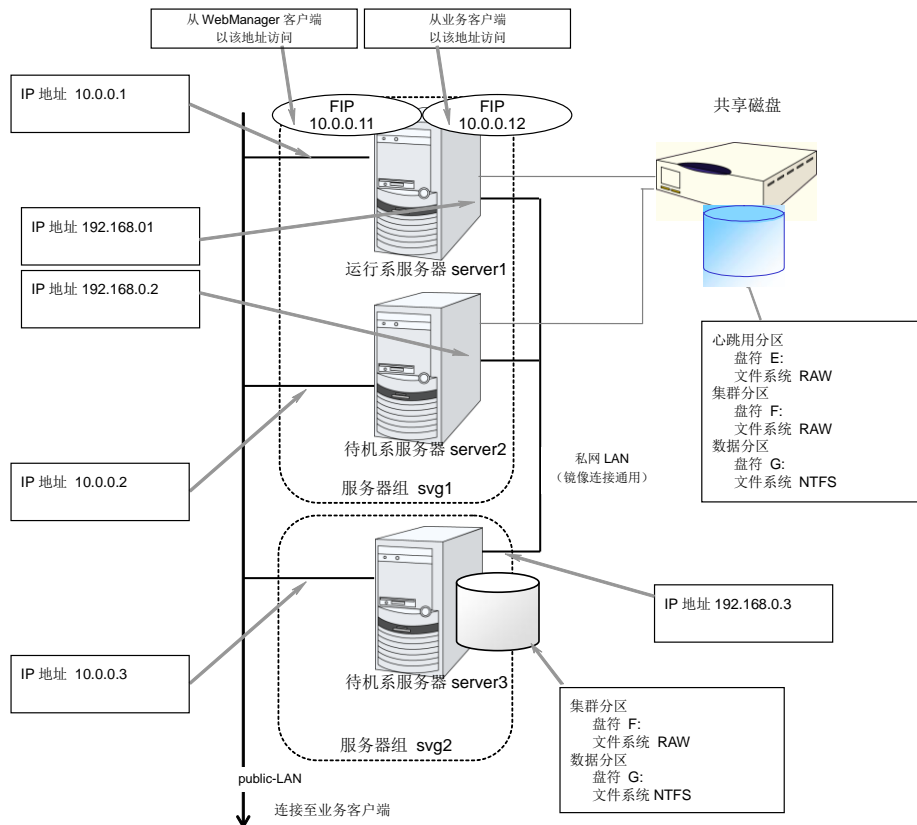
图 2-7 使用共享磁盘时的集群环境示例
