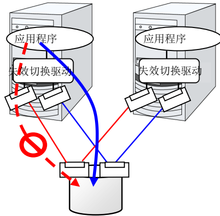
图 1-14 路径失效切换驱动
