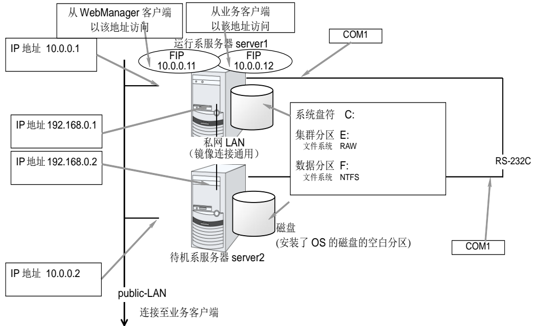
图 2-5 使用镜像磁盘时的集群环境示例
