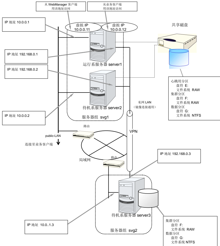
图 2-8 使用共享磁盘时的远程集群环境的示例
