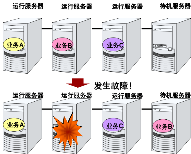
图 1-9 N + N 结构
